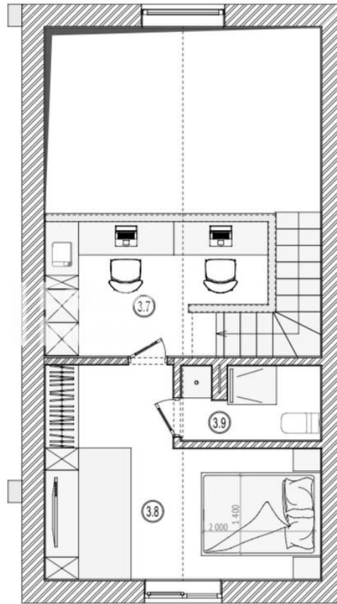
2-й этаж
