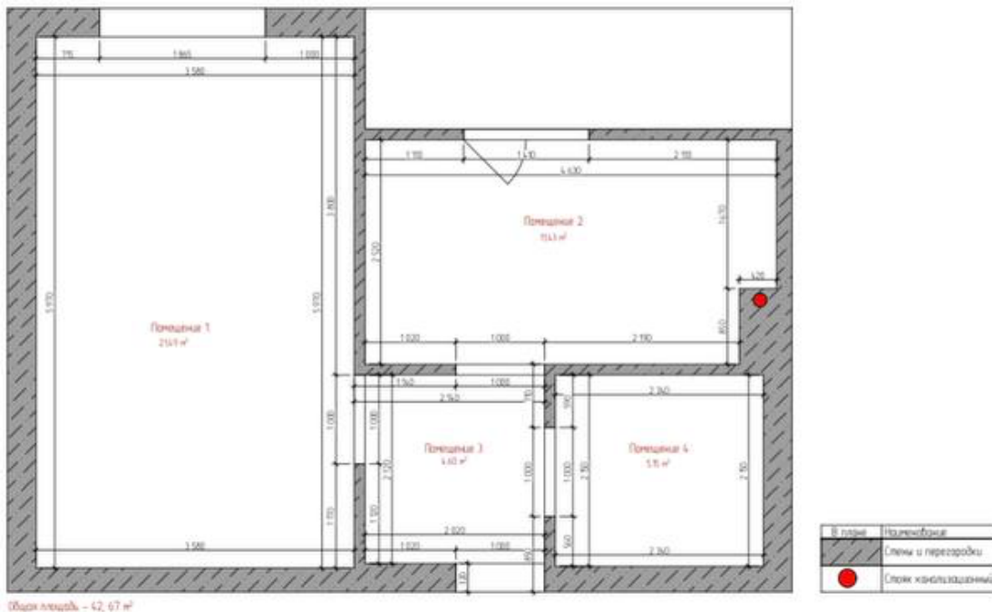
Обмерный план помещения.
